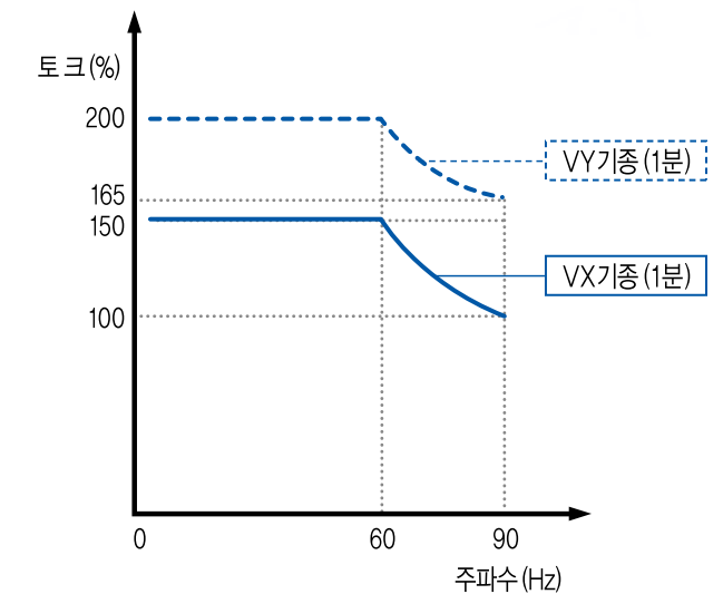
2.단시간 운전 토크 영역비교
